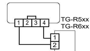
Schéma 2 : Raccordement de la sonde d'ambiance TG-R5xx ou TG-R6xx en cas de fonctionnement avec une consigne interne
