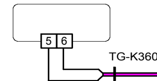
Abb. 7: Anschluss des Begrenzungsfühlers
