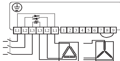
Schéma 1 : Raccordement de la tension d'alimentation et de la charge
