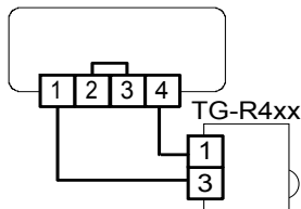
Abb. 3: Anschluss des TG-R430 als externer Fühler und Sollwertversteller bei Raumregelung.
