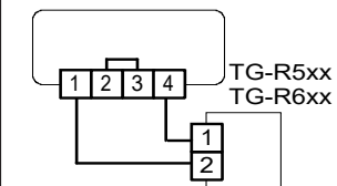
Figur 2: Inkoppling av rumsgivare TG-R5xx eller TG-R6xx vid drift med internt börvärde
