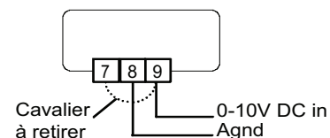
Schéma 8 : Raccordement pour un signal de commande externe
