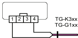
Abb. 4: Anschluss eines Fußboden oder Kanalfühlers bei Verwendung des internen Sollwertes.
