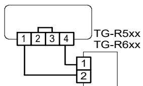
Abb. 2: Anschluss des Raumtemperaturfühlers TG-R5xx oder TG-R6xx bei Verwendung des internen Sollwertes
