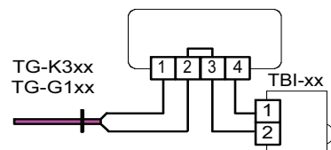
Figur 6: Inkoppling vid extern, separat givare och potentiometer TBI-xx som börvärdesinställning
