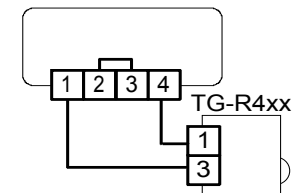
Schéma 3 : Raccordement de la sonde d'ambiance externe TG-R430 et réglage de consigne en ambiance.
