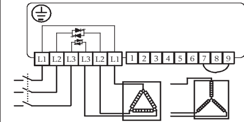
Figur 1: Inkoppling av matningsspänning och belastning
