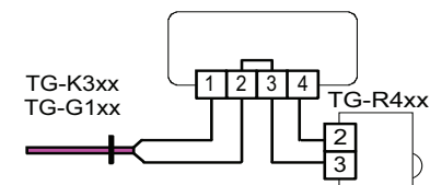
Schéma 5 : Raccordement en cas de sonde séparée externe et d'une TG-R4xx comme réglage de consigne seulement.
