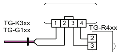
Abb. 5: Anschluss eines externen, separaten Fühlers und TG-R4XX lediglich als Sollwertversteller
