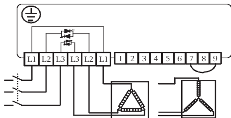
Abb. 1: Anschluss der Versorgungsspannung und Last
