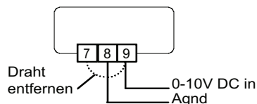
Abb. 8: Anschluss bei externem Stellsignal
