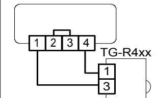
Figur 3: Inkoppling vid rumsreglering med TG-R430 som extern givare och börvärdesinställning
