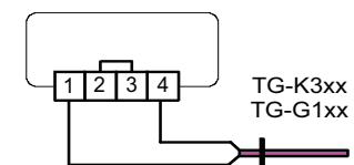
Schéma 4 : Raccordement des sondes de gaine et de sol en cas de fonctionnement avec une consigne interne
