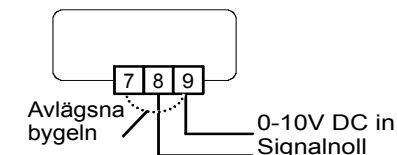
Figur 8: Inkoppling av extern styrsignal
