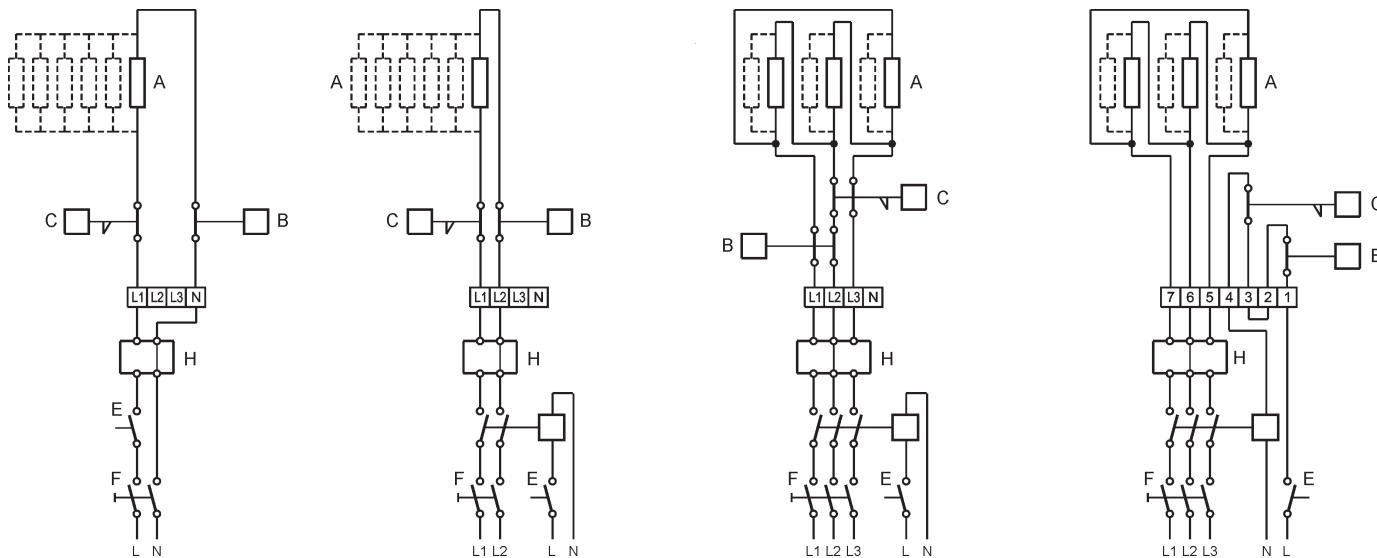
CB-1 (230V~)
